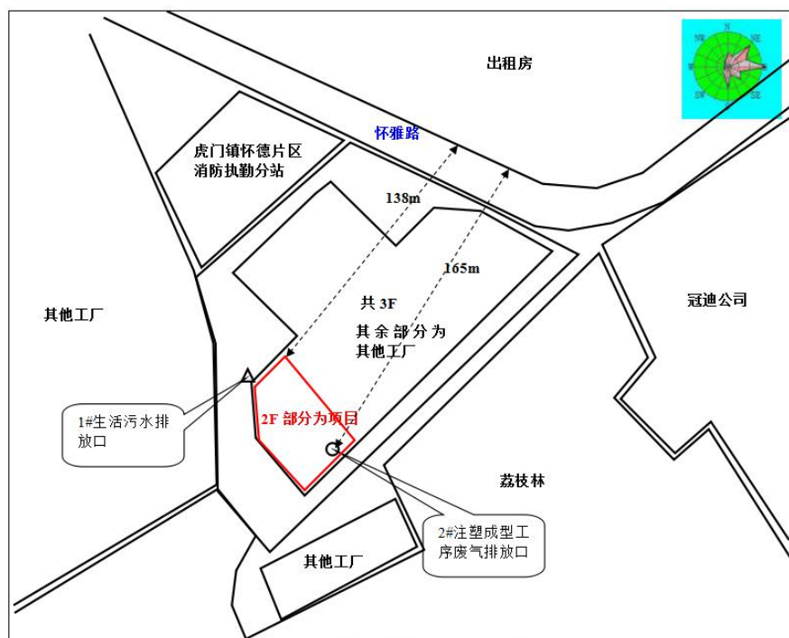
图3-1 厂区平面布置及监测点位
