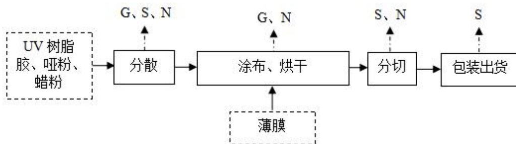
图 3-3 项目防刮哑膜的生产工艺及产污环节流程图
